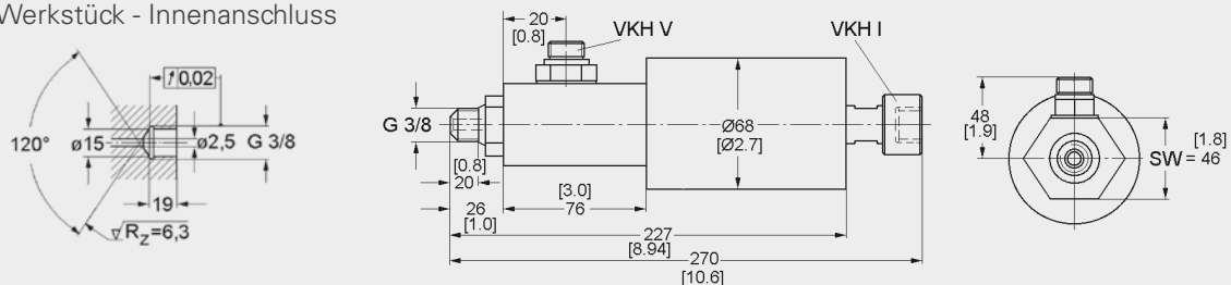
Werkstück - Innenanschluss
